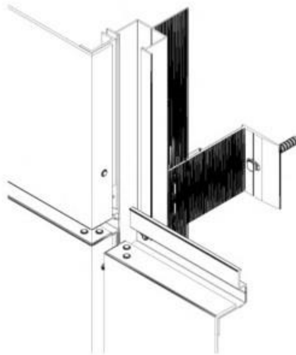
KOMPOZITNI PANEL A-2 COMPOSITE PANEL A-2
